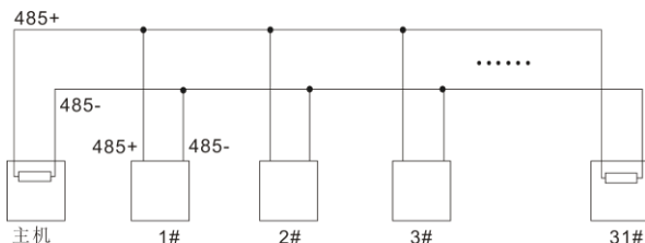
图 B-1 菊花接法现场接线图
