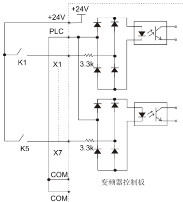
图3-13 干接点共阳极接线示意图
