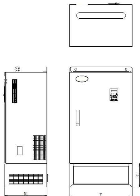
图 2-7-1：底座安装示意图
