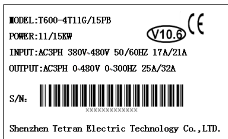
图 2-2 铭牌
